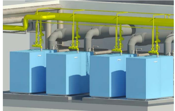
BIM model – napojenie kotolne
