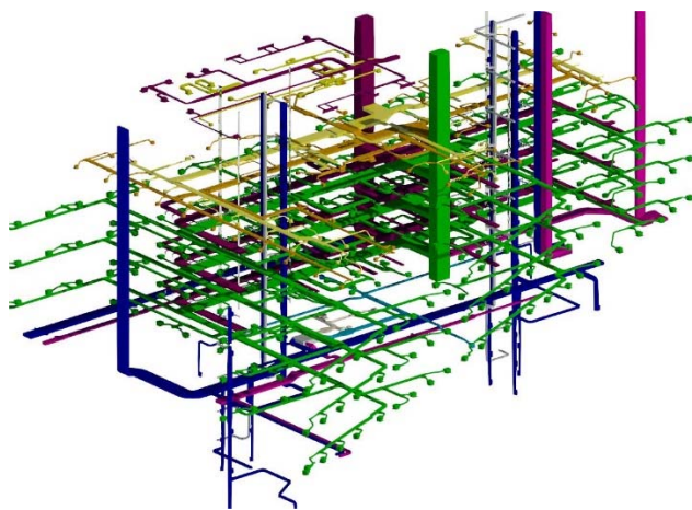
Riešenie rozvodov VZT
