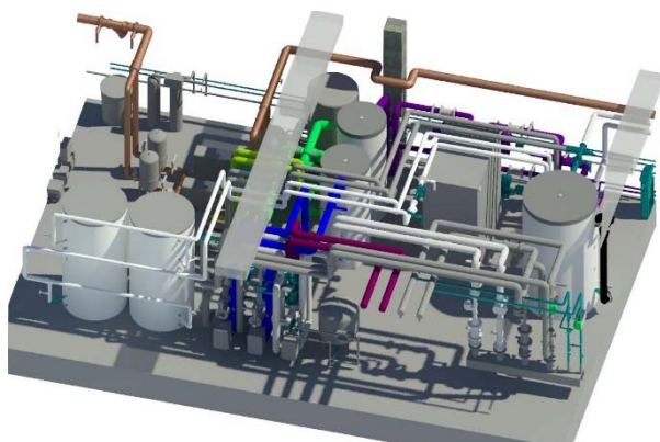
Riešenie zdroja vykurovania a chladenia
